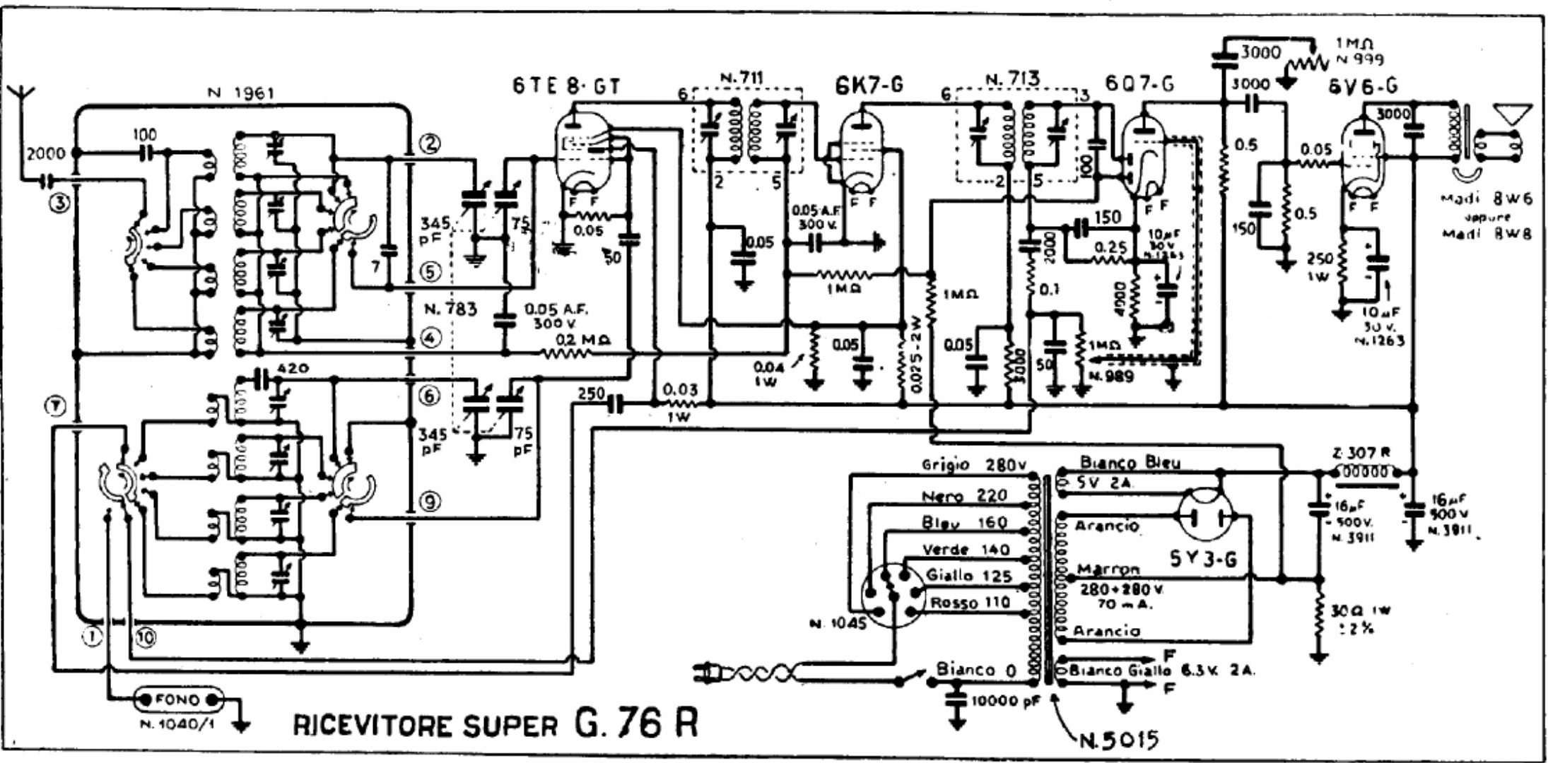
GELOSO (SOC.) - MOD. SUPER « G 76 R » (6TE8-GT)
